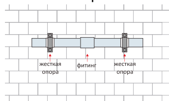
Крепление с двумя жесткими опорами и фитингом между ними
