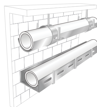
Установка трубопровода в свободном желобе
