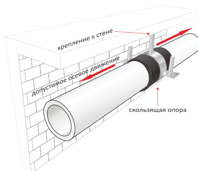
Установка со скользящими опорами
