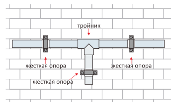
Крепление при разведении тройником
