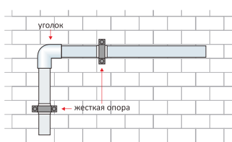
Крепление при разведении углом
