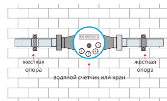
Крепление водяного счетчика или крана
